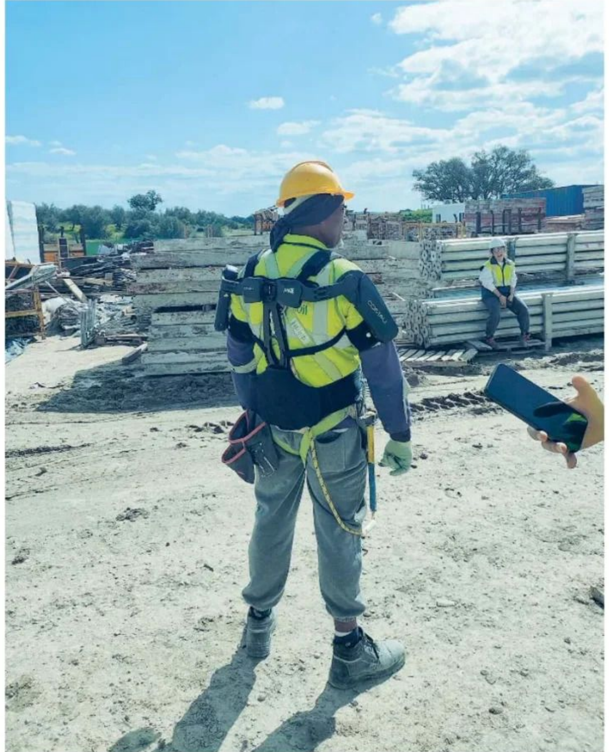
Exoesqueleto testado por Acciona en las obras de construcción del Hospital del Alentejo, Portugal
